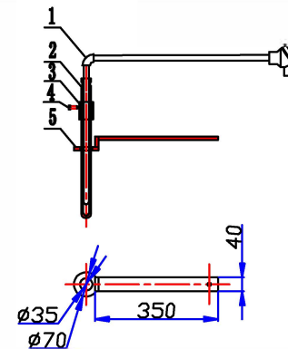
坩埚炉铝液温针配Φ28氮化硅保护套图示意
